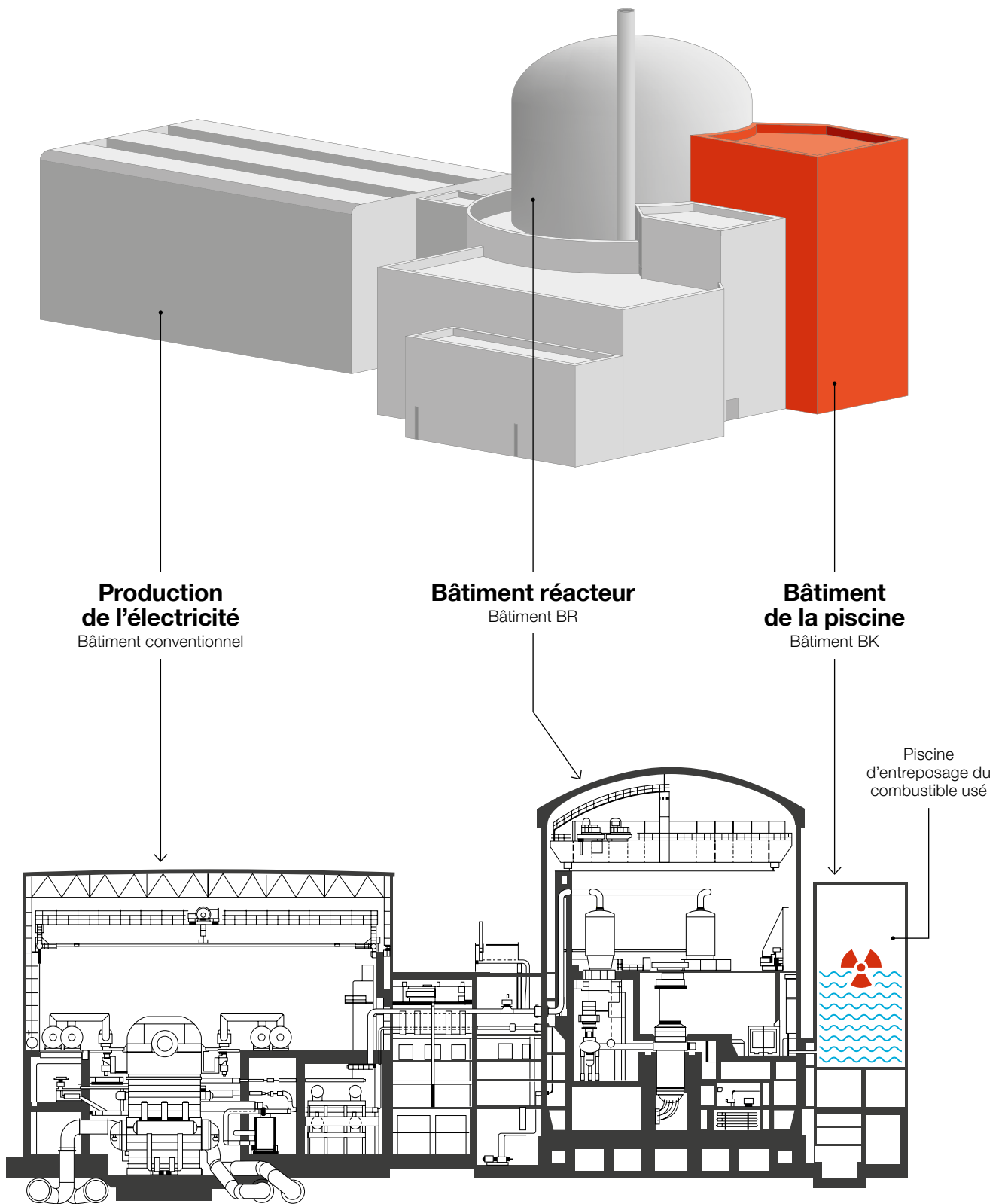
Coupe transversale d'une centrale nucléaire de production d'électricité
